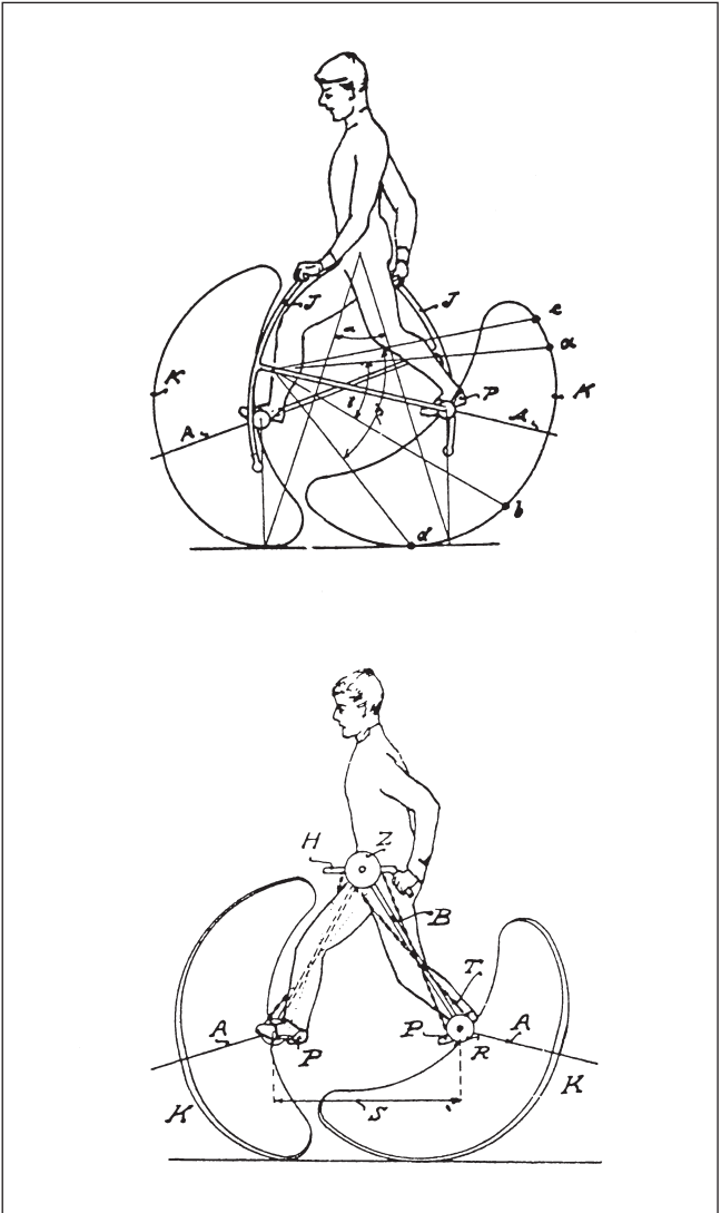
Resim 4: Robert Michael'in viraj ayakkabısı (1903) adımı büyültmek için bir Mekanizma (DRP 152 505).
