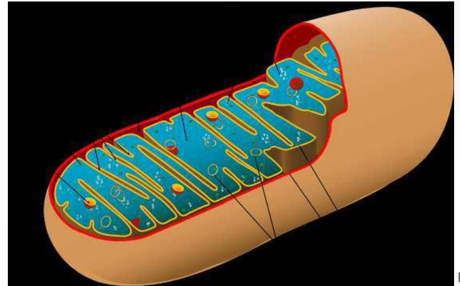
mtDNA
